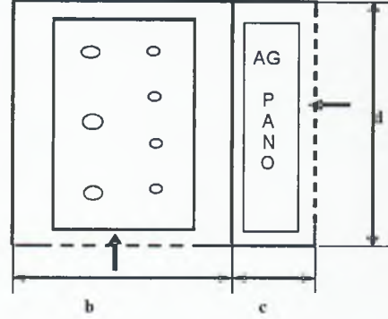
YG/AG TRANSFORMATÖR+AG PANO BÖLÜMÜ (TİP 2T)
