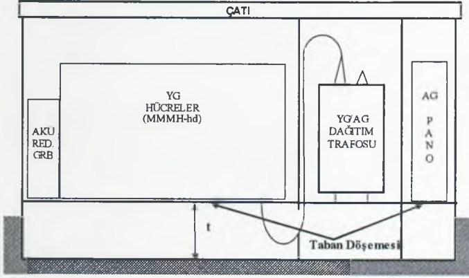
TİP-1 TEK PARÇALI, İÇERİDEN İŞLETİLEN TİP KOMPAKT MERKEZ (max.1600 kVA),
