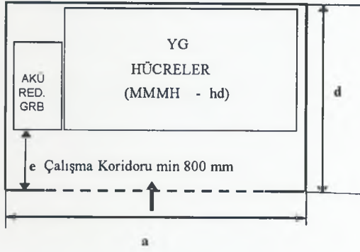
YG HÜCRE BÖLÜMÜ (TİP-2H/A-D)
