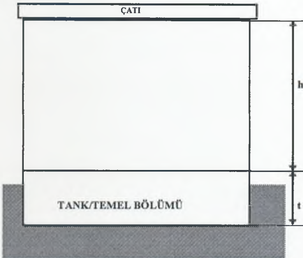
YG HÜCRE BÖLÜMÜ (TİP-2H/A-D)
